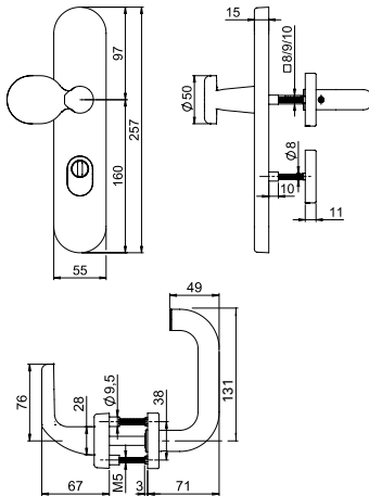
G-160 / D-110
