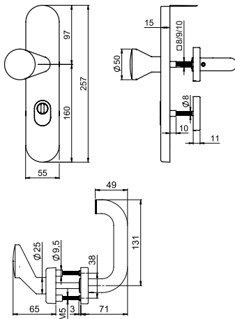
G-150 / D-110
