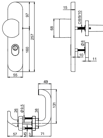
G-180 / D-110
