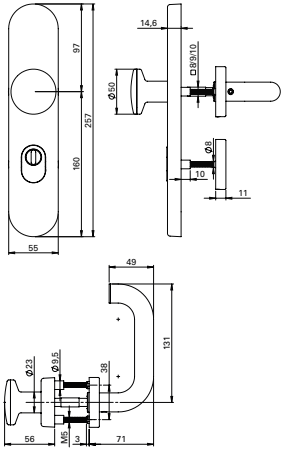
K-130 / D-110
