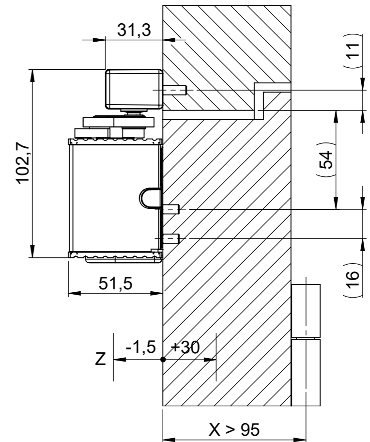
A-A (1 : 2)
