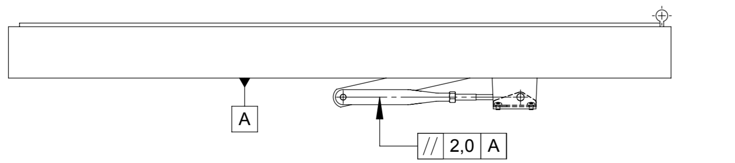
Anbauvariante Montageplatte + Scherengestänge (SGS)
