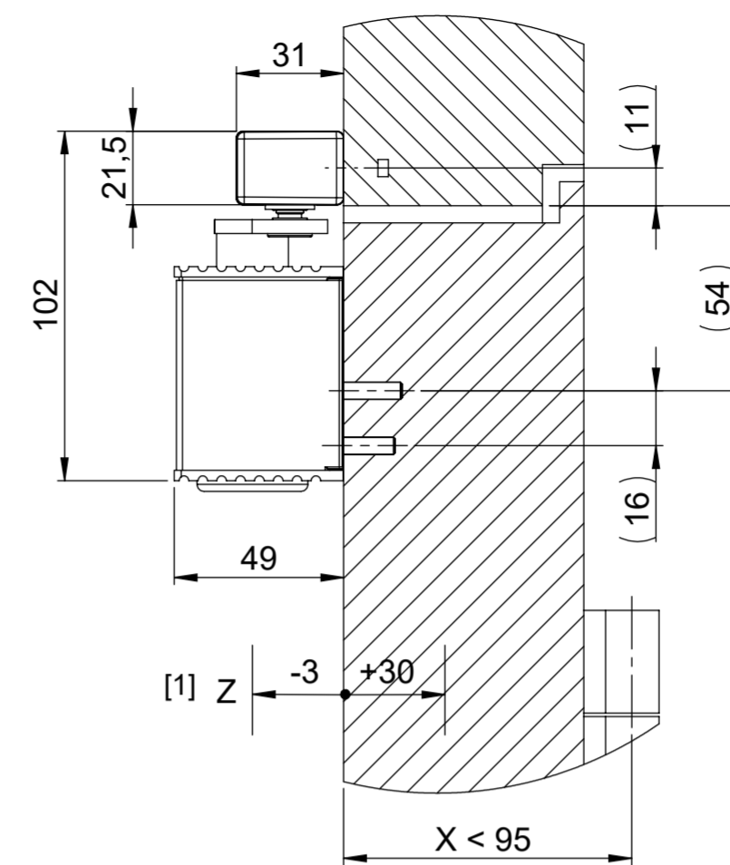
[1] Maximaler Überstand für überstehende Zargen (Z = positiv) und überstehende Türblätter (Z = negativ)
