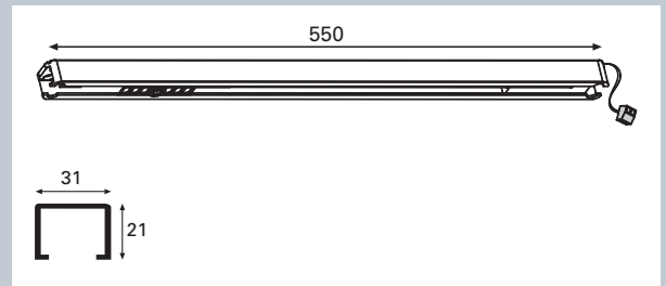
Montage de la glissière ECO IS EF
