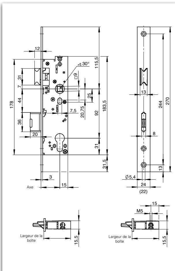
Dimensions : GBS 97
