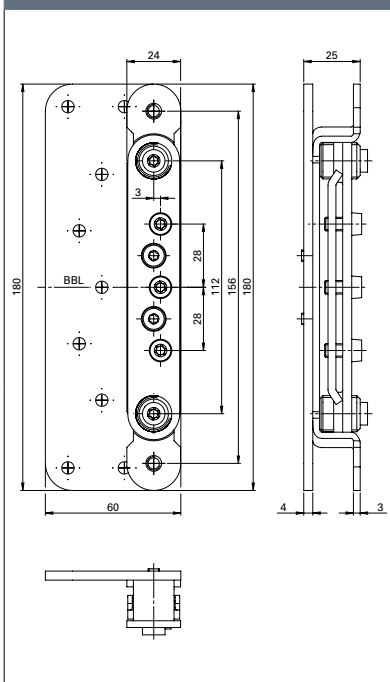
Schéma des dimensions
