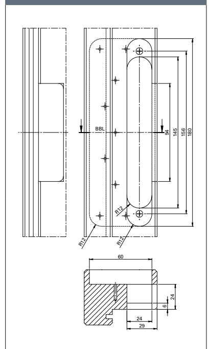
Schéma de fraisage avec angle de recouvrement
