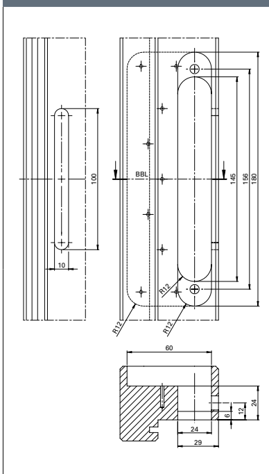
Schéma de fraisage avec tôle de recouvrement
