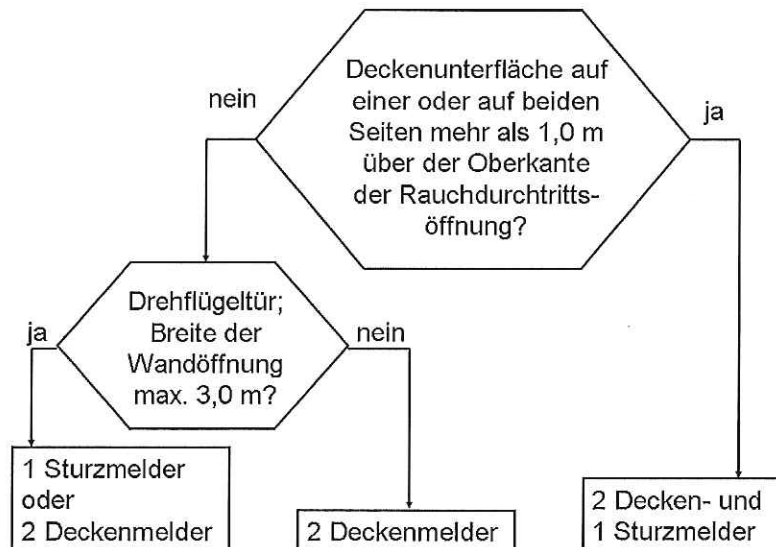
Bild 3: Entscheidungsdiagramm
